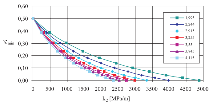
Rys. 4. Wartości \kappa_{\min} dla górotworu o współczynniku zwięzłości f = 3,5 (wytrobiska korytarzowe łukowe)
