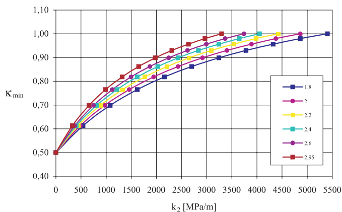
Rys. 5. Wartości \kappa_{\max} dla górotworu o współczynniku zwięzłości f = 3,5 (wytrobiska korytarzowe kołowe)
