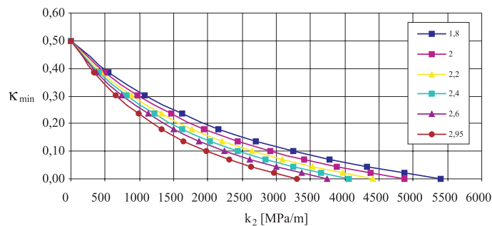
Rys. 3. Wartości \kappa_{\min} dla górotworu o współczynniku zwięzłości f = 3,5 (wytrobiska korytarzowe kołowe)
