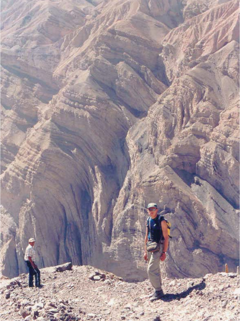
Fig. 5. Sfałdowane utwory mezozoiczne w Kanionie Colca poniżej Ayo
