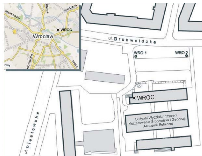
Rys. 1. Lokalizacja permanentnej stacji GPS/GLONASS na terenie Wrocławia
