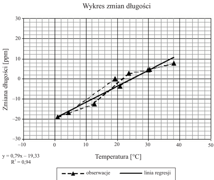
Rys. 6. Względne zmiany długości wstęgi inwarowej w czasie wyznaczania WLRT (Leica 27119) – po stabilizacji
