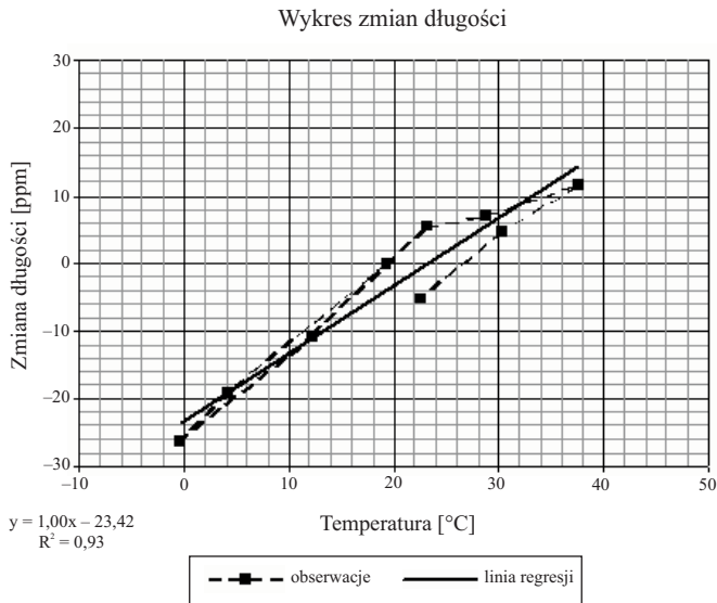
Rys. 5. Względne zmiany długości wstęgi inwarowej w czasie wyznaczania WLRT (Leica 27119) – przed stabilizacją
