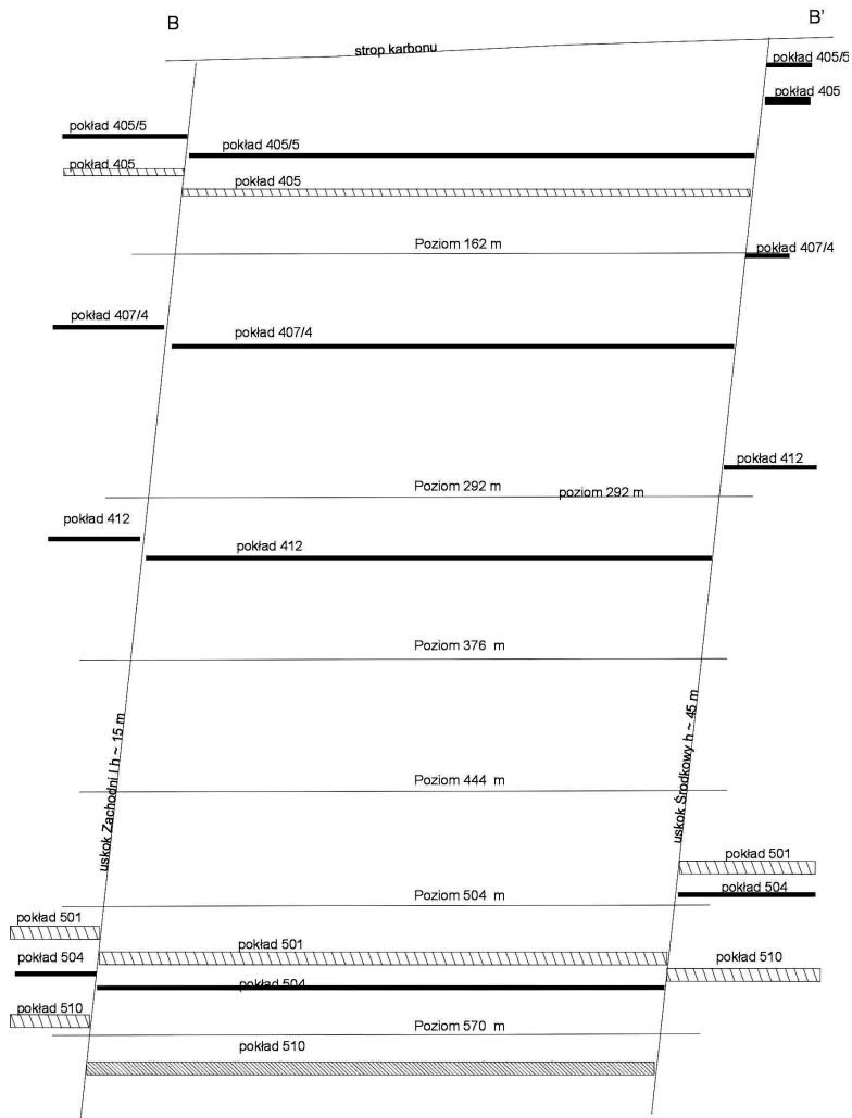
Rys. 3. Schemat warunków górnictwo-geologicznych w rejonie składowiska w zrobach pokładu 510 [9]
