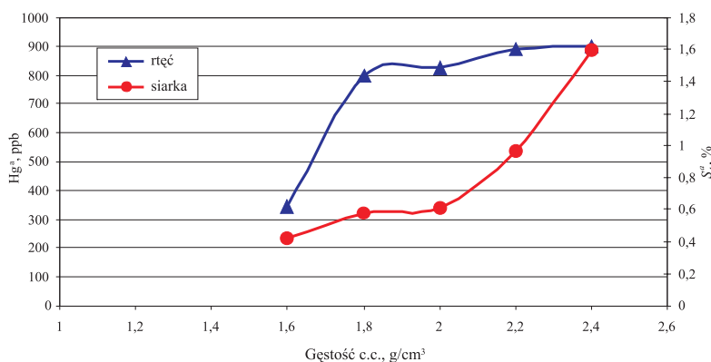
Rys. 10. Zawartość rtęci i siarki całkowitej w poszczególnych frakcjach węgla o uziarnieniu 0,04÷0,5 mm
