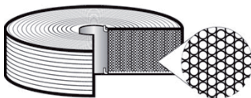
Rys. 4. Przekrój zbiornika rurek [10]
