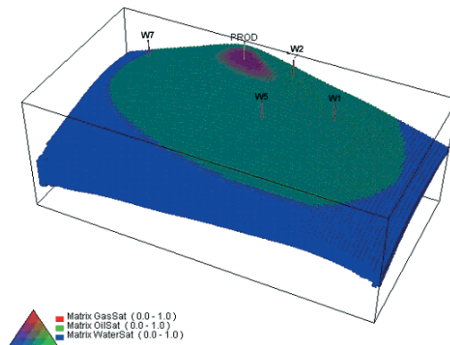
Rys. 2. Nasycecie płynami złożowymi przed rozpoczęciem eksploatacji odwiertem multilateralnym
