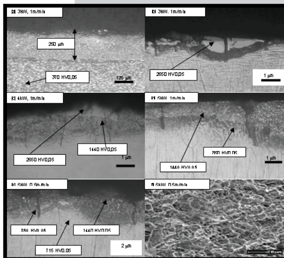
RYS.1. Przykładowe mikrostruktury przekrojów i mikrotwardość warstwy nadtopionej (a-e) oraz przełom (SEM) strefy przypowierzchniowej warstwy nadtapianej (f).
