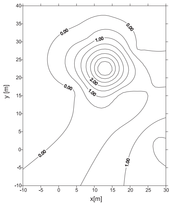
Rys. 7. Ekwiwalentna koncentracja propanu w gazach gruntowych [% obj.] na głębokości 1,2 m ppt
