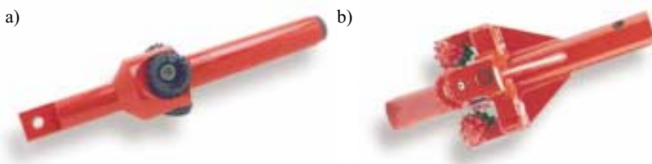
Rys. 7. Rozwiertaki rolkowe: a) Rockmaster; b) Rhino Rock [3]
