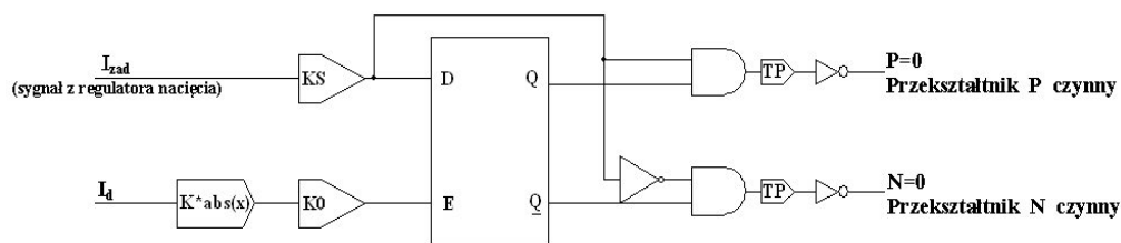
Rys. 7. Schemat blokowy układu blokady wyzwalania impulsów załączających przekształtników
