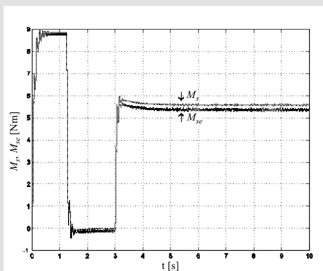
Rys. 7. Przebiegi rzeczywistego M_s oraz estymowanego M_{se} momentu skracajacego układu napędowego przy J_1 < J_2
