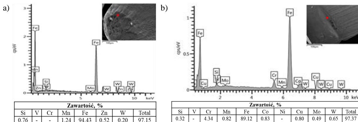
Rys. 8. Widmo charakterystycznego promieniowania rentgenowskiego z obszaru śladu zużycia ostrza skrawającego po toczeniu z chłodziwem zawierającym: a) asparaginian cynku, b) olej mineralny
