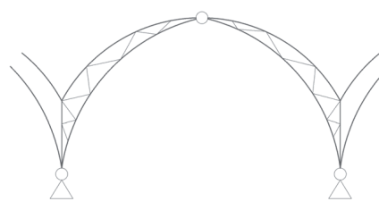
Fig. 4. Milano Centrale (1931)
