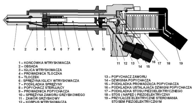
Rys. 8. Schemat piezoelektrycznego wtryskiwacza Continental – Siemens
