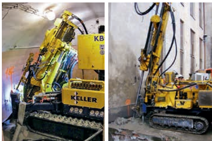
Ryc. 17 i 18. Wiertnica podczas pracy: (po lewej) wiertnica KB-0 podczas pracy na zewnątrz budynku, (po prawej) wiertnica KB-1 podczas pracy w piwnicach budynku
