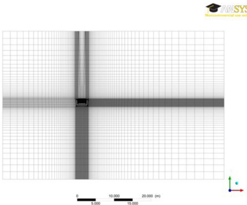
Rys. 2. Siatka objętości skończonych zastosowana w analizie opływu
