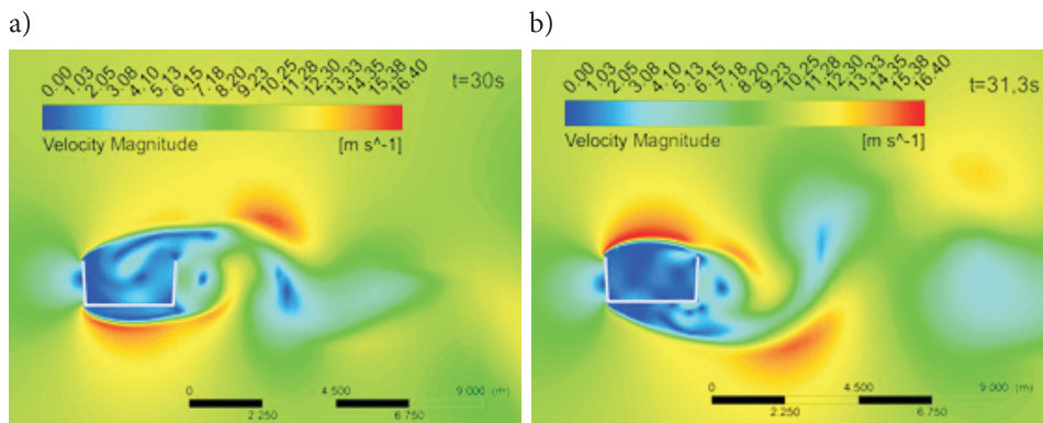
Rys. 3. Mapa wypadkowej wektora prędkości — ślad wirowy, w t = 30 s (a) i w t = 31,3 s (b)
