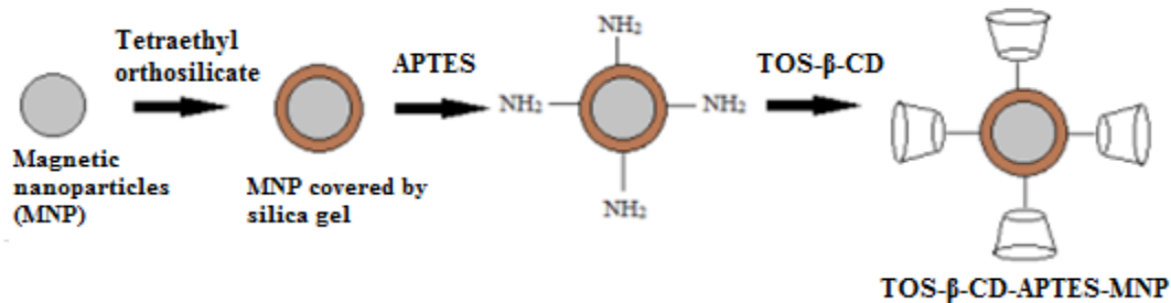
Fig. 4. Modification schema.
