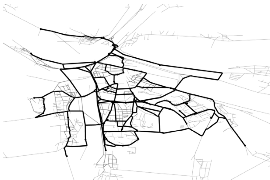
Fig. 2. Reduced transportation network from problem with 200 relations Bild 2. Reduziertes Verkehrsnetz für das Problem mit 200 Relationen
