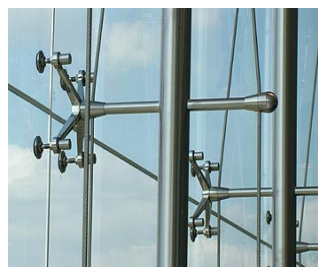
Ryc. 10. System strukturalny, sworzniowy (uchwyt typu plannar wall). Źródło: www.faraone.it
