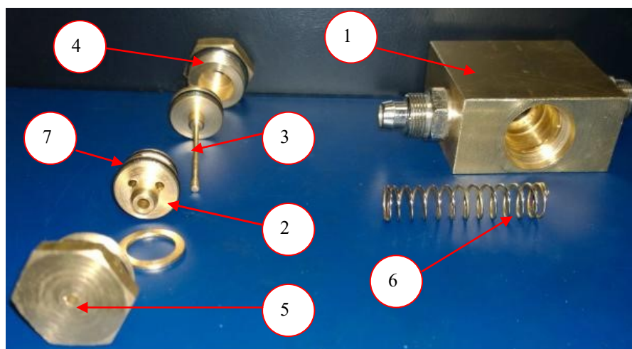
Rys. 2. Egzemplarz badawczy dyszy samoczyszczącej drobnokroplistej [11, 12]: 1 - korpus, przyłączeniowy, 2 - dysza wewnętrzna, 3 - iglica z tłoczkiem, 4 - tuleja wylotowa, 5 - korek zamykający, 6 - sprężyna, 7 - uszczelnienia
