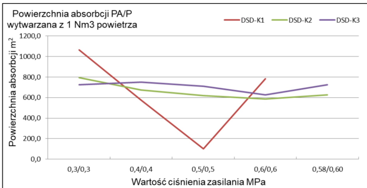
Rys. 11. Powierzchnia absorpcji PA/P w zależności od ciśnienia mediów zasilających [12]
