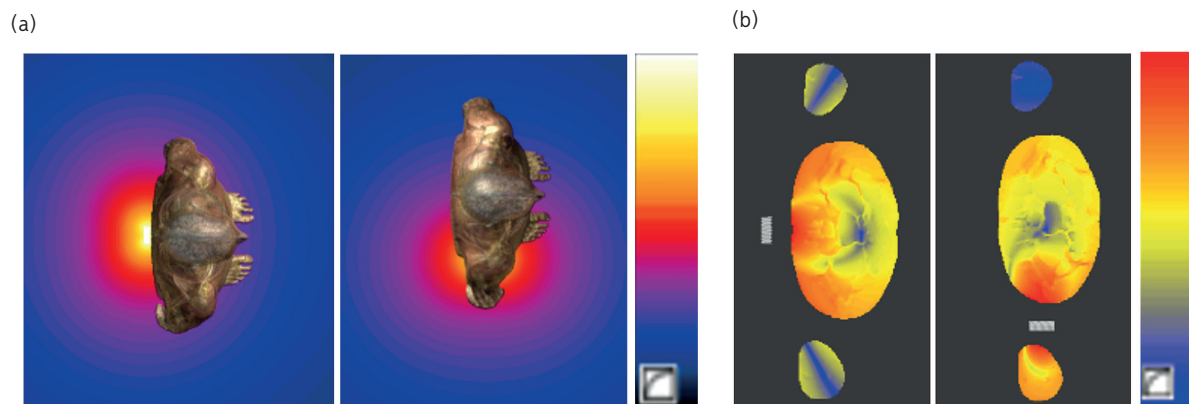
Rycina 3. Przykładowe rozkłady natężenia pola magnetycznego przy lokalizatorze (a) oraz natężenia pola elektrycznego indukowanego w ciele jego użytkownika (b); lokalizator emitujący pole-EM o częstotliwości 250 kHz, umieszczony za plecami (po lewej stronie) lub z boku użytkownika (po prawej stronie)
