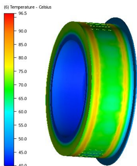
Rys. 4. Wyniki obliczeń termicznych przy stałej prędkości pojazdu 50\text{ km/h} po nachyleniu powierzchni 20\% , przy temperaturach początkowych jak na rysunkach 2 i 3 i przepływie chłodziwa 15\text{ l/min} a) wirnik b) stojan
