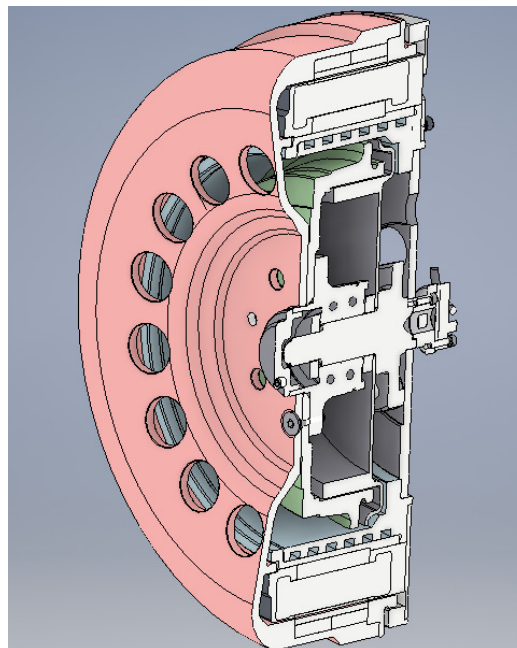
Rys. 1. Model 3D przekroju silnika
