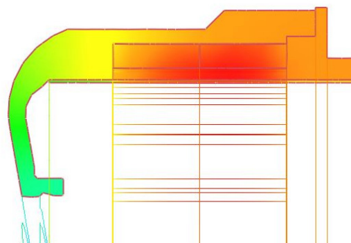
Rys. 3. Wyniki obliczeń termicznych przy stałej prędkości pojazdu 150 \text{ km/h} po nachyleniu powierzchni 0\% i przepływie chłodziwa 15 \text{ l/min} a) wirnik b) przekrój wirnika
