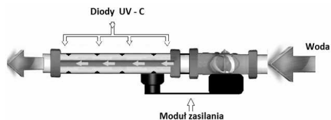
Rys. 8. Koncepcja układu wspomagającego dezynfekcji wody
