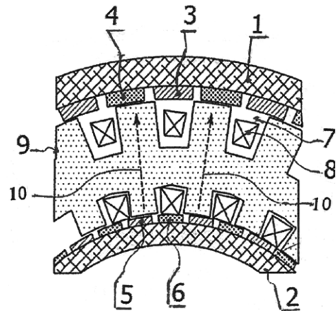
Rys. 2. Przykład rozwiązania obwodu magnetycznego i uzwojeń maszyny scalonej: 1 - wirnik zewnętrzny; 2 - wirnik wewnętrzny; 3, 5 - magnesy N; 4, 6 - magnesy S; 7 - żłobki; 8 - uzwojenie; 9 - jarzmo twornika; 10 - indukcja
