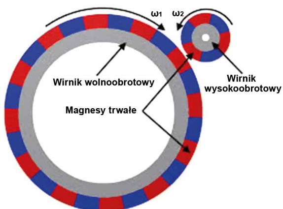
Rys. 3. Przekładnia magnetyczna modelująca przekładnię mechaniczną [3, 4]
