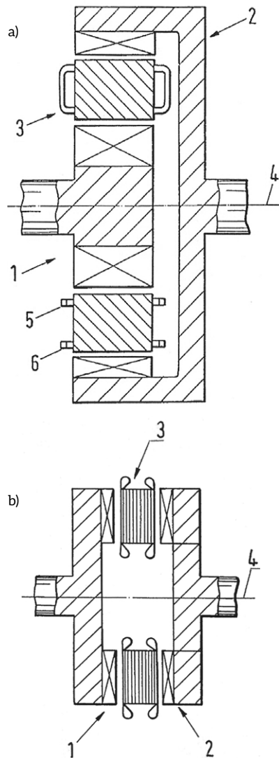
Rys. 1. Scalona konstrukcja dwóch maszyn elektrycznych: a) rozwiązanie cylindryczne; b) rozwiązanie tarczowe. Oznaczenia: 1 - wirnik wewnętrzny; 2 - wirnik zewnętrzny; 3 - twornik; 4 - oś wałów; 5, 6 - uzwojenia twornika [2]
