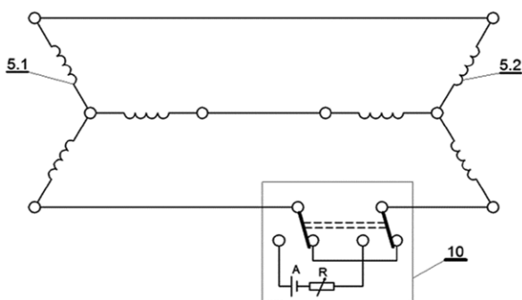
Rys. 7. Schemat połączenia jednej fazy uzwojeń z przełącznikiem trójbiegunowym i ze źródłem napięcia stałego
