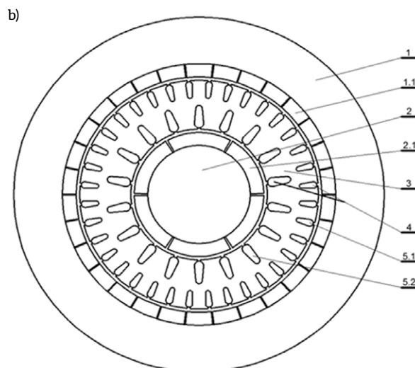
Rys. 4. Przekładnia magnetyczna: a) przekrój wzdłużny; b) przekrój poprzeczny obwodu magnetycznego przekładni
