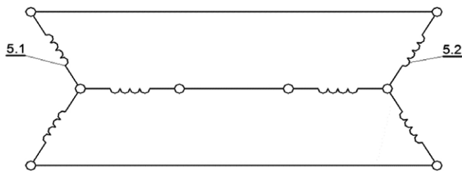
Rys. 5. Schemat połączenia uzwojeń przy pracy jednokierunkowej przekładni
