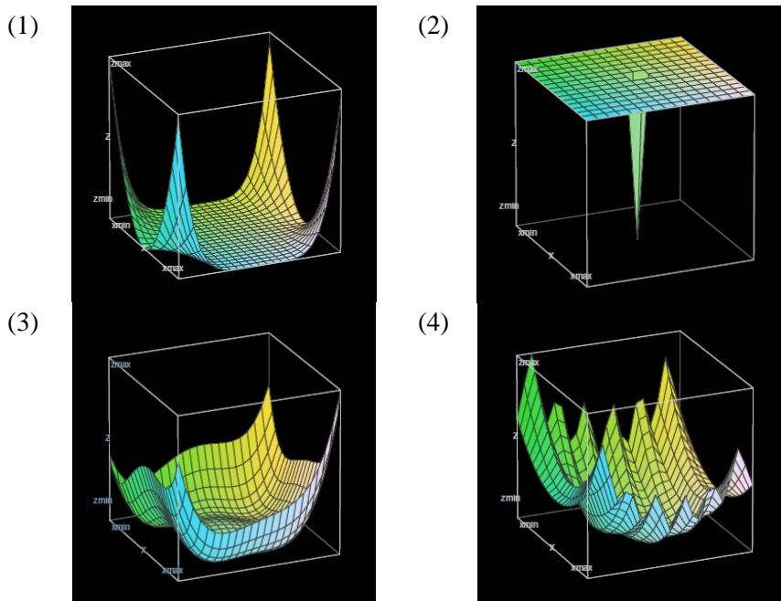
Rysunek 1. Wizualizacje funkcji (1) Beale'a (2) Easoma, (3) Himmelblau , (4) Levy'ego.
