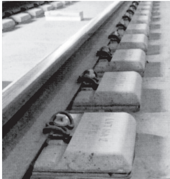
Rys. 5. Widok nawierzchni kolejowej LVT ułożonej w torach tunelu św. Gotarda
