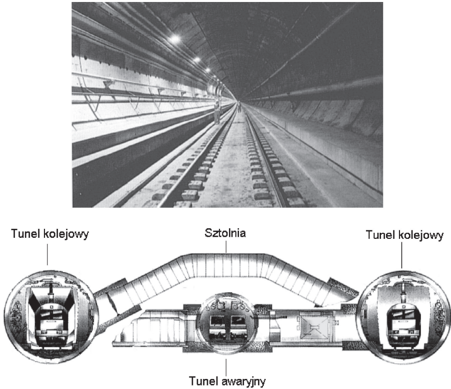
Rys. 1. Widok tunelu pod kanałem La Manche i jego przekrój poprzeczny
