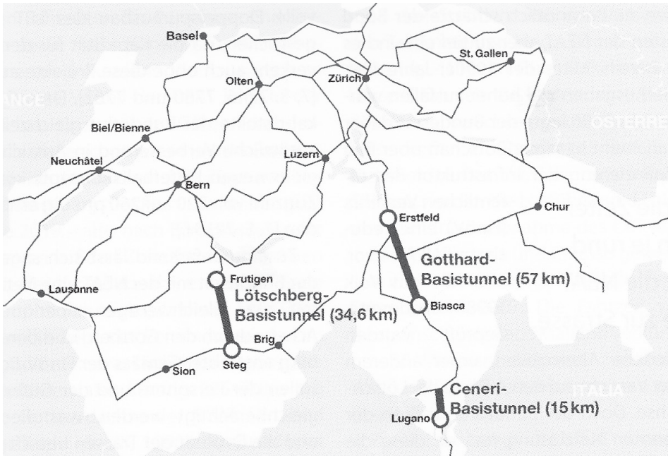
Rys. 3. Tunel św. Gotarda jako element kolejowego przejścia przez Alpy
