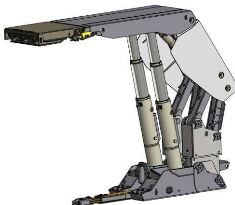
Rys. 12. Model komputerowy sekcji obudowy HYDROMEL-29/46-POz/BSN [9]
