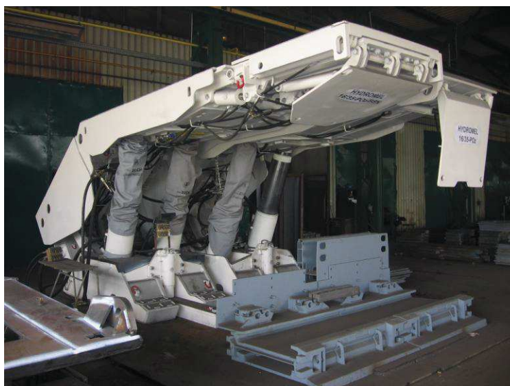
Rys. 5. Prototypy sekcji obudowy HYDROMEL-16/35-POz i HYDROMEL-16/35-POz/BSN w siedzibie Przedsiębiorstwa HYDROMEL S.A. [1]
