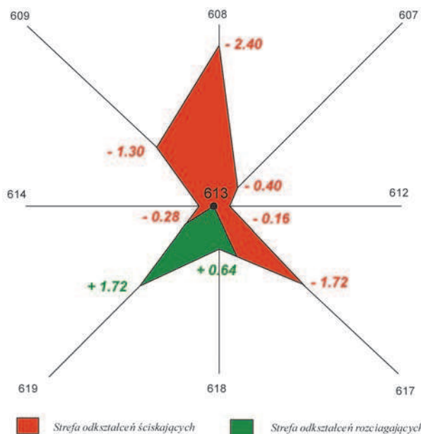
Rys. 3. Schemat powierzchniowego rozkładu odkształceń poziomych w granicach rozety „600” mniejszej (wewnętrznej)
