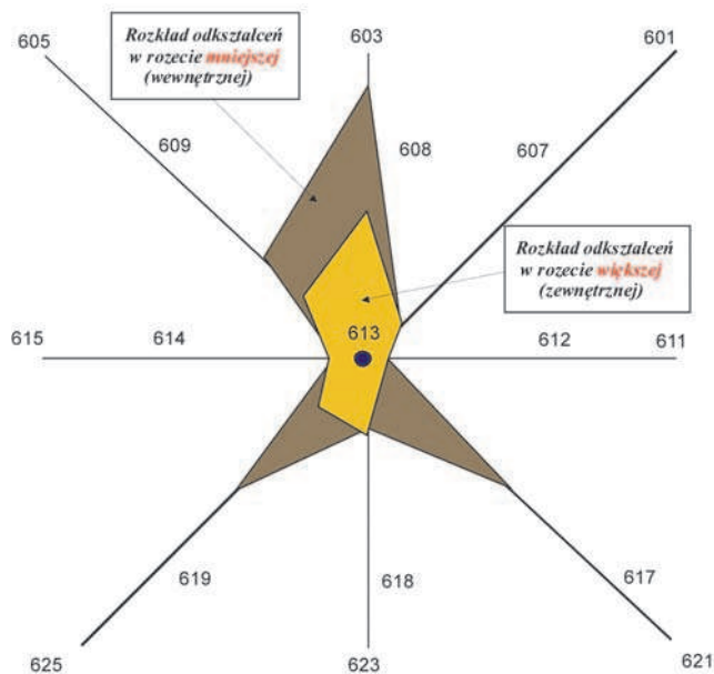
Rys. 4. Porównanie rozkładów odkształceń poziomych w granicach większej („zewewnętrznej”) i mniejszej („wewnętrznej”) rozety „600”
