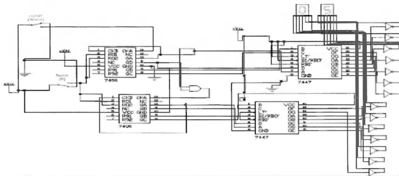
Rys 5. Schemat układu liczącego opracowanego w programie Electronics Workbench
