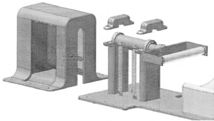
Rys. 11. Mechanizm urządzenia
