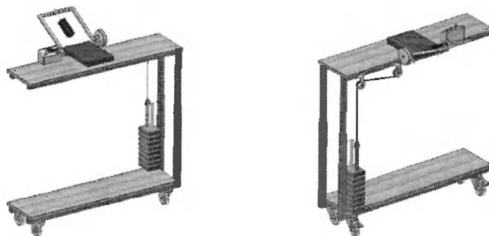
Rys. 2. Wirtualny model urządzenia po modernizacji
