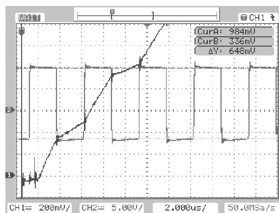
Rys. 3. Oscylogram przedstawiający zasadę działania układu pomiarowego.
