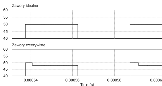
Rys. 1. Zniekształcenia napięcia wyjściowego falownika spowodowane spadkami napięcia na kluczach
