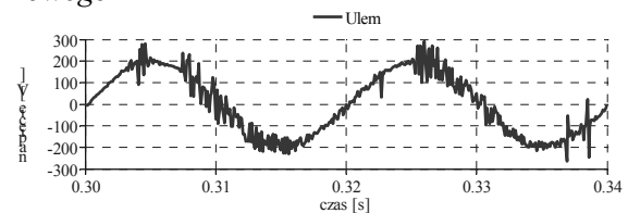
Rys. 8. Przebieg napięcia wyjściowego falownika uzyskany z zewnętrznego przetwornika typu LEM podłączonego do wyjść falownika poprzez filtr dolnoprzepustowego
