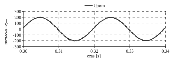
Rys. 9. Przebieg napięcia wyjściowego falownika uzyskany z układu pomiaru napięcia wyjściowego
