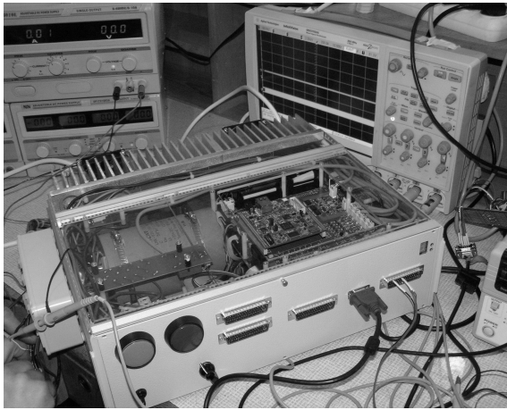
Rys. 4. Zdjęcie falownika
