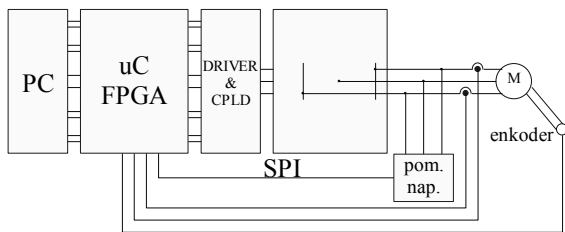
Rys. 5. Struktura Schemat blokowy całego falownika.
