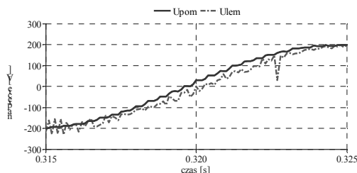
Rys. 10. Porównanie przebiegu napięcia wyjściowego falownika uzyskanego z zewnętrznego przetwornika typu LEM podłączonego do wyjść falownika poprzez filtr dolnoprzepustowy z przebiegiem napięcia wyjściowego falownika uzyskanego z układu pomiaru napięcia wyjściowego
