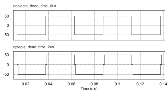
Rys. 2. Zniekształcenia napięcia wyjściowego falownika wywołane czasem martwym
