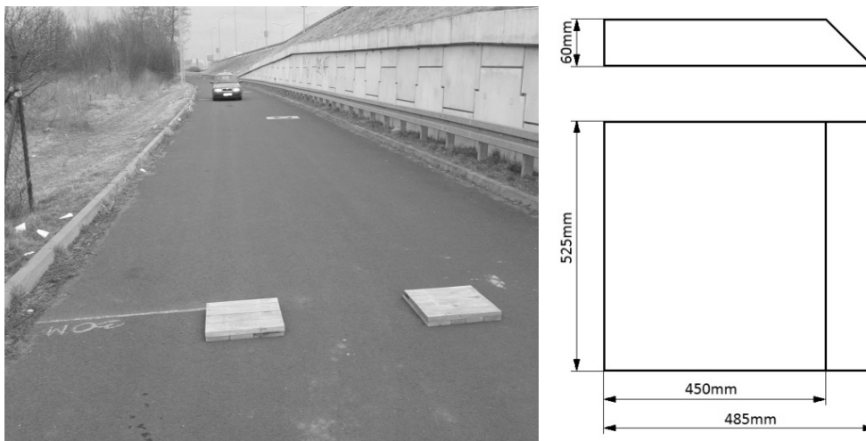
Fig. 3. View of the roadblock on the route (left photo), the dimensions of the roadblock (right picture) Rys. 3. Widok przeszkody stałej na drodze (po lewej), wymiary przeszkody (po prawej)
