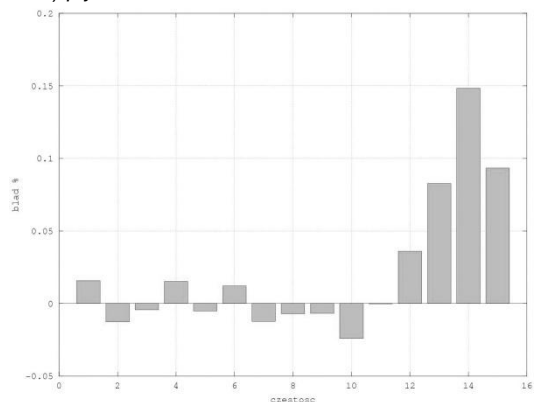
Rys. 2. Wartości błędów przy wyznaczaniu wartości własnych płyt
