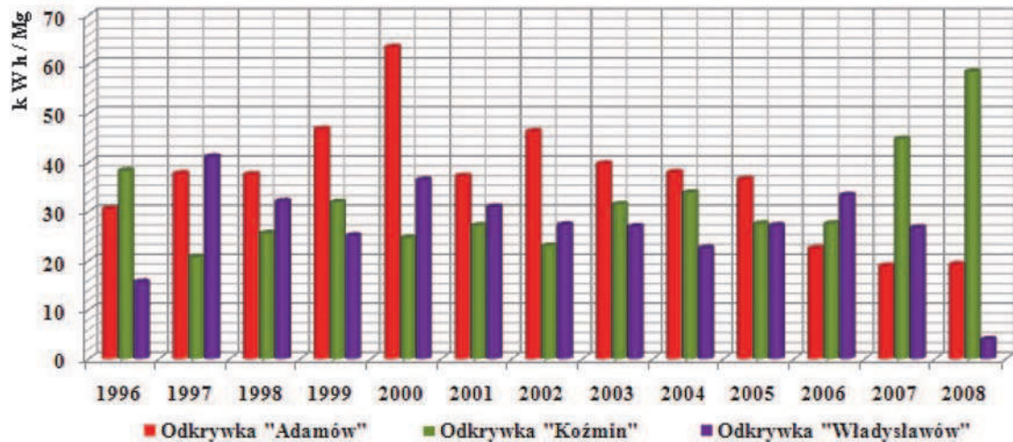
Ryc. 6. Zużycie energii elektrycznej na 1 Mg węgla w poszczególnych odkrywkach KWB „Adamów” w latach 1996 – 2008
