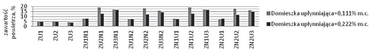
Rys. 1. Wyniki badań zaprawy wzorcowej
