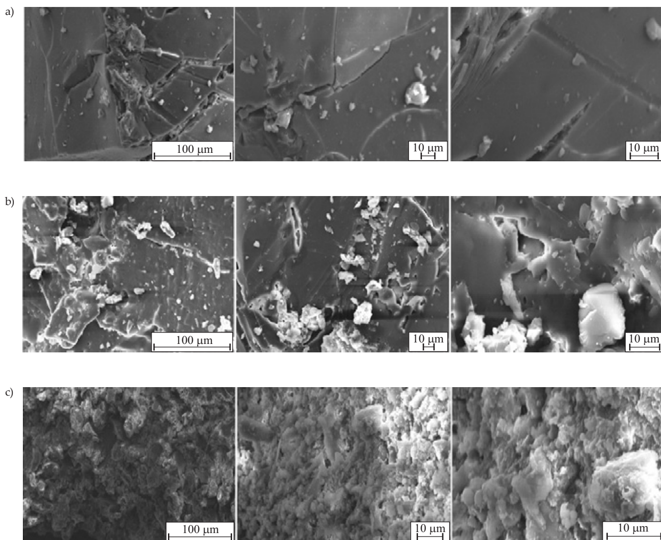
Fig. 9. SEM images of: a) P-2HBA, b) P-2HBA3MP, and c) P-2HBATAP
