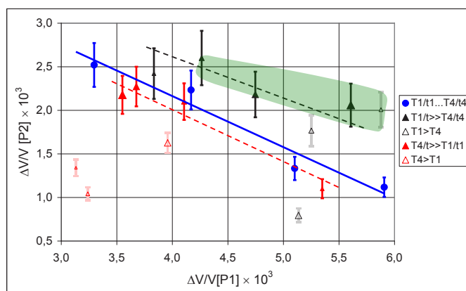
Rys. 6. Zależność względnej zmiany objętości towarzyszącej procesowi P2 od zmiany objętości towarzyszącej procesowi P1; obróbka standardowa (T1/t1...T4/t4), dwustopniowa (>>) oraz nagrzewanie lub studzenie (>) z szybkościami q = 1,2 i 4 K/min
