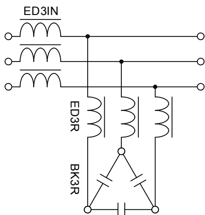
Rys. 2. Schemat obwodowy filtra harmonicznego ElhandHF
