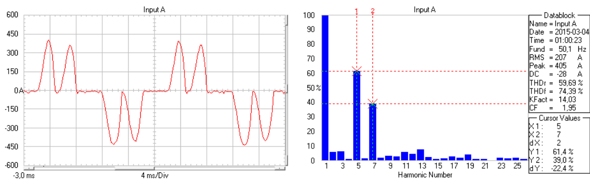
Rys. 8a. Oscylogramy prądu wejściowego przekształtnika przy 1% efektywnej impedancji
