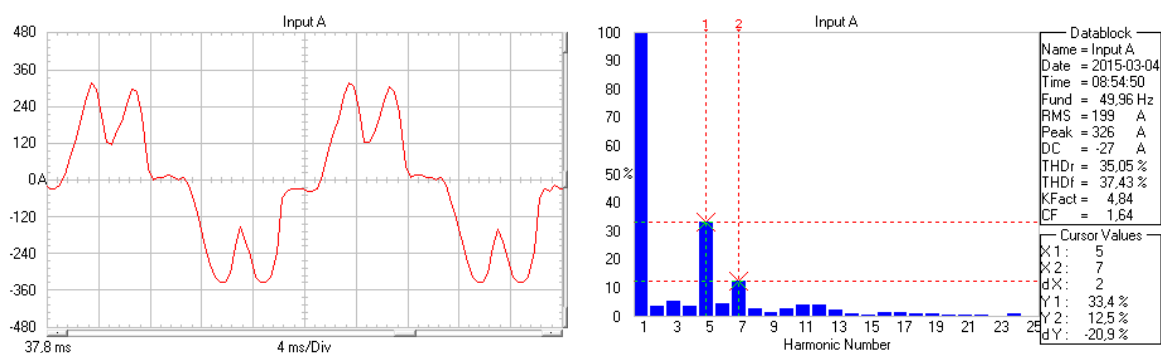
Rys. 8b. Oscylogramy prądu wejściowego przekształtnika przy 5% efektywnej impedancji
