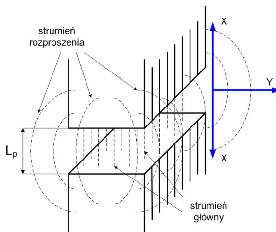
Rys. 4. Strumień główny i rozproszenia w obszarze przyszczelinowym
