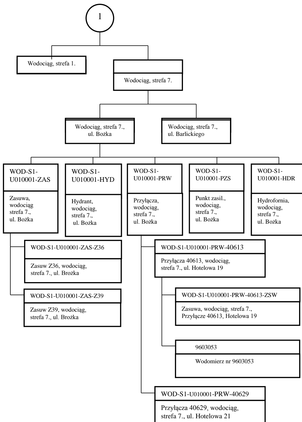
Rys. 4. Fragment struktury obiektów technicznych PWiK
