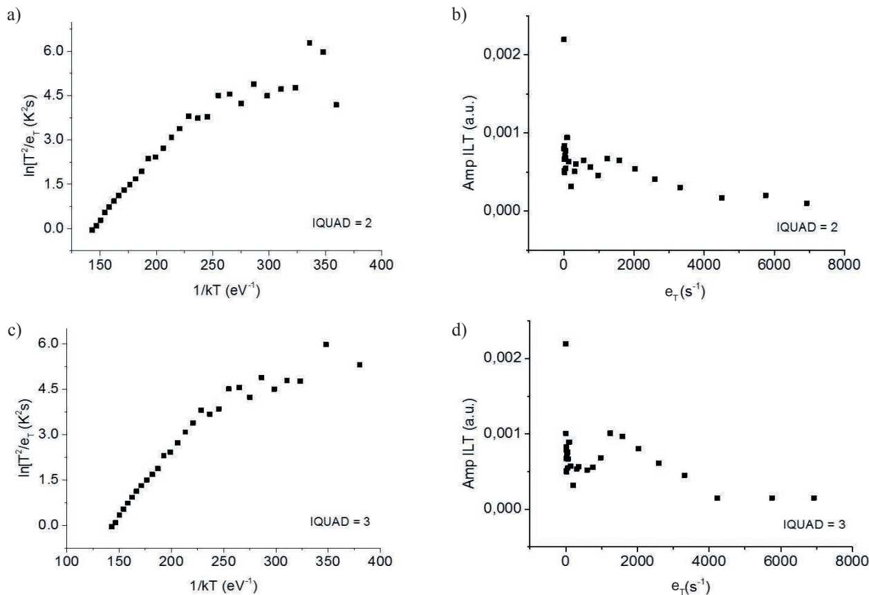
Rys. 9. Zilustrowanie wpływu wartości parametru IQAD programu CONTIN na układ punktów tworzących wykresy Arrheniusa (a, c) oraz układ punktów tworzących zależności wysokości linii grzbietowej fałdy w dwuwymiarowym widmie Laplace'a od szybkości emisji (b, d).
