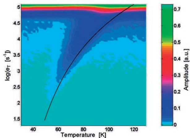
Rys. 1. Korelacyjny prążek widmowy dla radiacyjnych centrów defektowych wykrytych w MCz-Si napromieniowanym neutronami o energii 1 MeV. Linia ciągła ilustruje temperaturową zależność szybkości emisji nośników ładunku dla centrów defektowych o energii aktywacji E_a = 0,047 eV i współczynniku A = 8,2 \times 10^2 s -1 K -2 .
