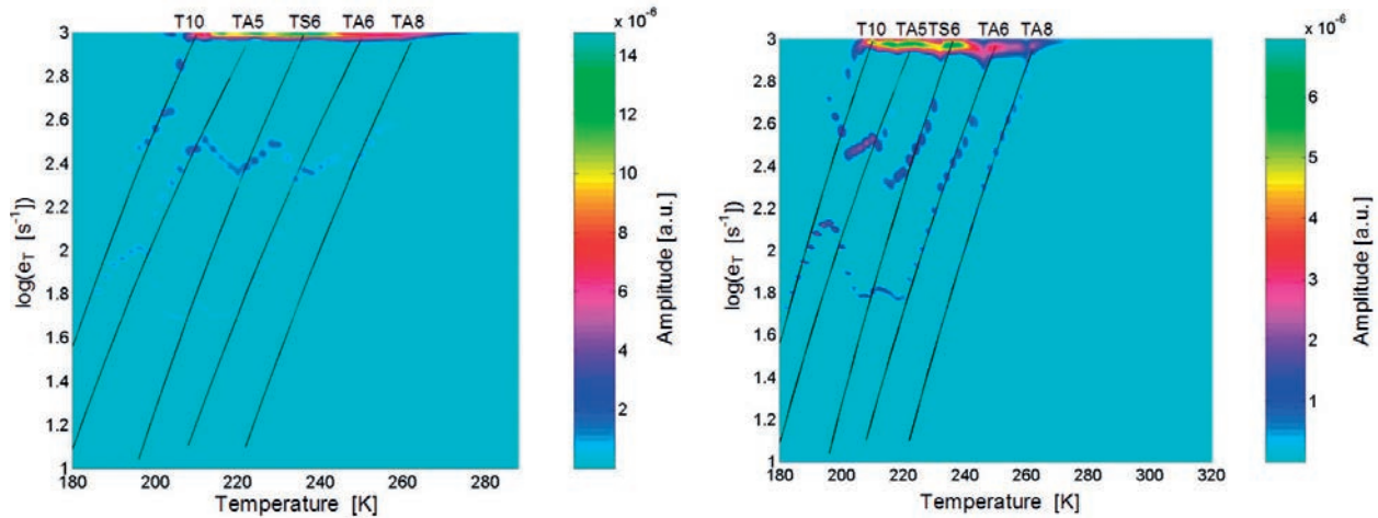
Rys. 15. Obraz prążków widmowych Laplace’a otrzymany na podstawie symulowanych relaksacyjnych przebiegów fotoprądu wywołanych termiczną emisją nośników ładunku z centrów defektowych T10, TA5, TS6, TA6 i TA8 z dodaną składową szumową. IWT = 2 (a) i IWT = 3 (b) oraz GMNMX2 = 1.E+3 (a, b), wartości pozostałych parametrów programu CONTIN takie jak na Rys. 2. Fig. 15. Image of the Laplace spectral fringes obtained from the simulated photocurrent relaxation waveforms related to the thermal emission of the charge carriers from the T10, TA5, TS6, TA6 and TA8 defect centers with an added noise component. IWT = 2 (a) and IWT = 3 (b) and GMNMX = 1.E+3 (a, b), the values of the remaining parameters are as in Fig. 2.
