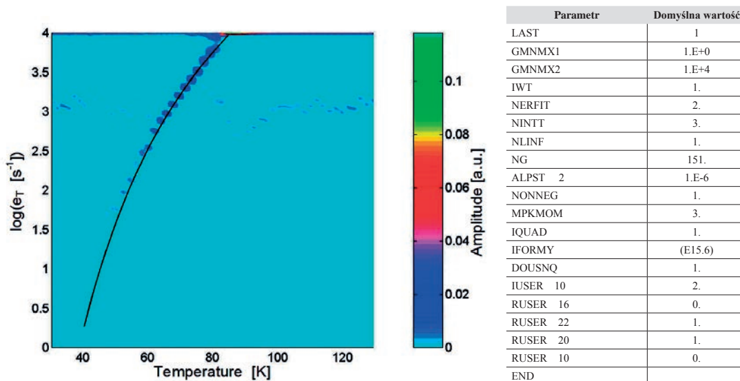
Rys. 2. Widmowy prążek Laplace’a uzyskany za pomocą programu CONTIN dla radiacyjnych centrów defektowych o energii aktywacji E_a = 0,047 eV i współczynnika A = 8,2 \times 10^2 s -1 K -2 . Linia ciągła ilustruje temperaturową zależność szybkości emisji nośników ładunku. W tabeli zestawiono wartości parametrów programu CONTIN, dla których wykonano obliczenia numeryczne w celu otrzymania prążka widmowego.
