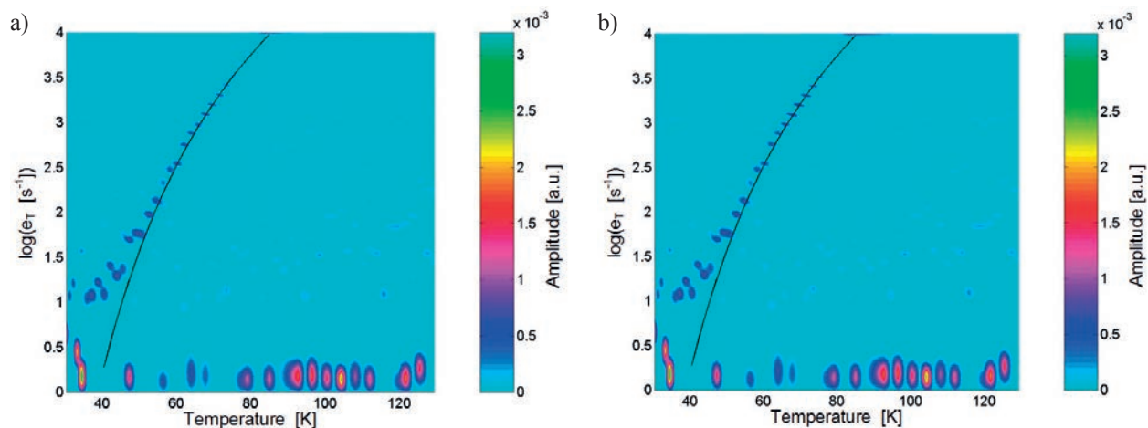
Rys. 8. Zilustrowanie wpływu parametru IQAD programu CONTIN na obraz prążka widmowego Laplace'a dla radiacyjnych centrów defektowych o energii aktywacji E_a = 0,047 eV i współczynnika A = 8,2 \times 10^2 s -1 K -2 . Wartości parametru IQAD są następujące: 2 (a) i 3 (b). Wartości pozostałych parametrów programu CONTIN takie jak na Rys. 2.
