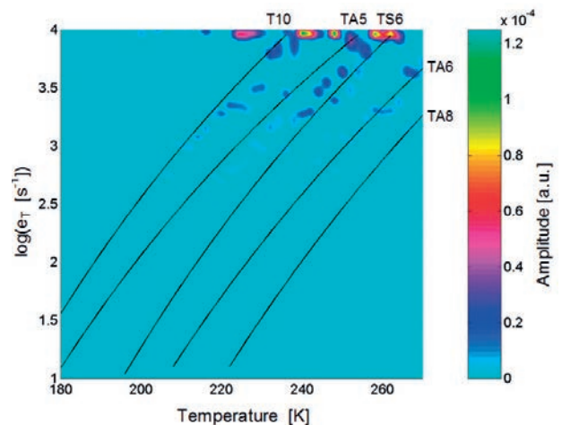
Rys. 14. Obraz prążków widmowych Laplace'a otrzymany na podstawie symulowanych relaksacyjnych przebiegów fotoprądu wywołanych termiczną emisją nośników ładunku z centrów defektowych T10, TA5, TS6, TA6 i TA8 z dodaną składową szumową.
