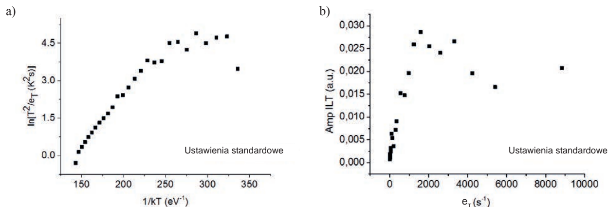
Rys. 3. Wykres Arrheniusa dla wykrytych centrów defektowych ( E_a = 0,047 eV, A = 8,2 \times 10^2 s -1 K -2 ) (a) oraz zależność wysokości linii grzbietowej fałdy w dwuwymiarowym widmie Laplace’a od termicznej szybkości emisji nośników ładunku (b).
