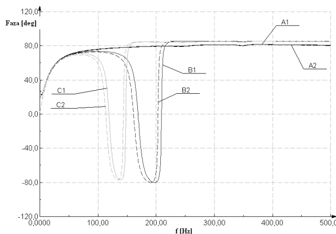
Rys. 3. Charakterystyki fazowe węzła PCC: kompensator SVC konfiguracja I; A – TSC wyłączony, B – załączona 1 sekcja TSC, C – załączone 2 sekcje TSC; 1 – największa wartość indukcyjności TCR ( B_{TCR} = \max lub B_{TCR} = -B_{TSC} ), 2 – TCR wyłączony ( B_{TCR} = 0 )
