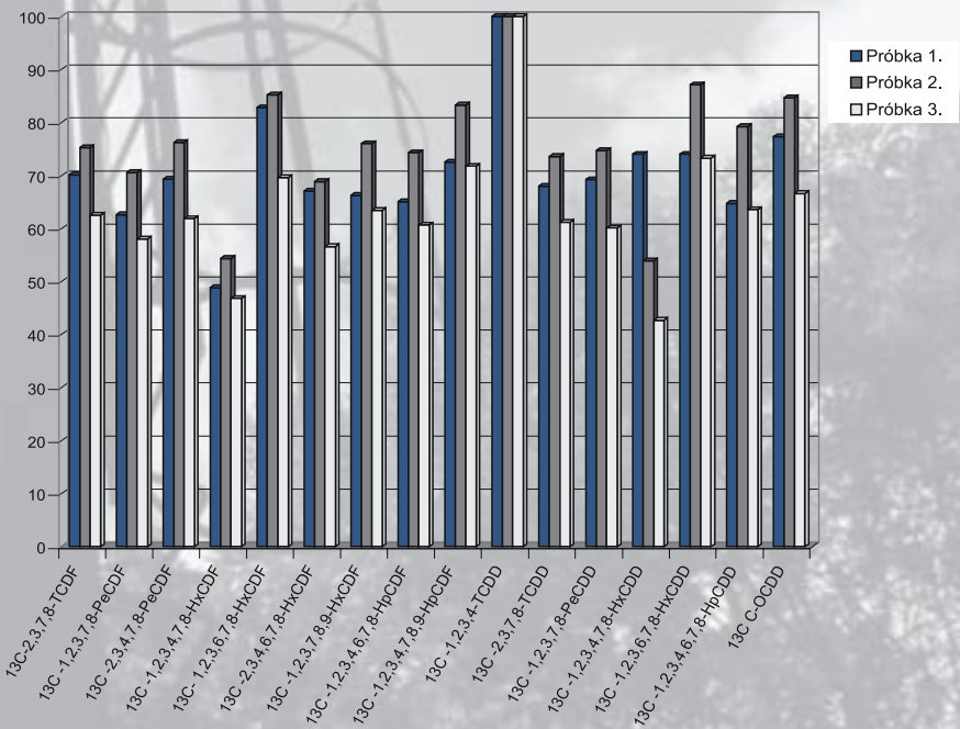
Rys. 2. Wartość odzysku dla wzorców wewnętrznych PCDDs/Fs znaczonej izotopowo węglem 13C Fig. 2. Recovery values of labelled PCDDs/Fs
