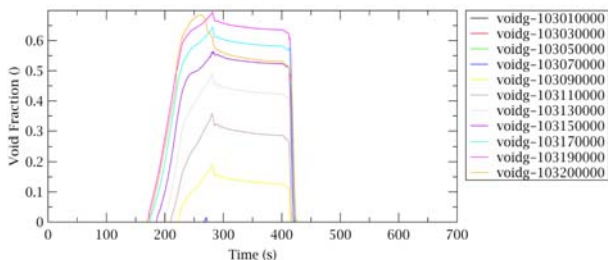
Fig. 17. Void fraction.
