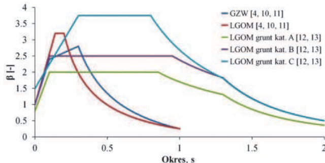
Rys. 7. Przyjęte wymuszenia kinematyczne w postaci przyspieszeniowych spektrów odpowiedzi
