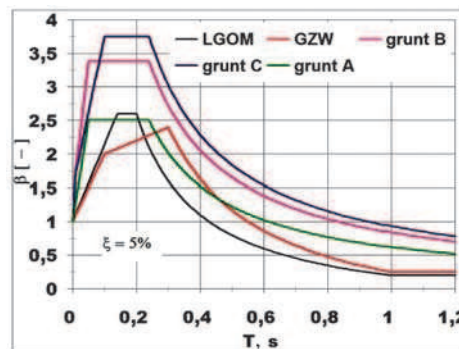
Rys. 8. Porównanie wzorcowych spektrów odpowiedzi dla obszarów GZW i LGOM ze spektrum wzorcowym typu 2 z EC 8 dla różnych warunków gruntowych
