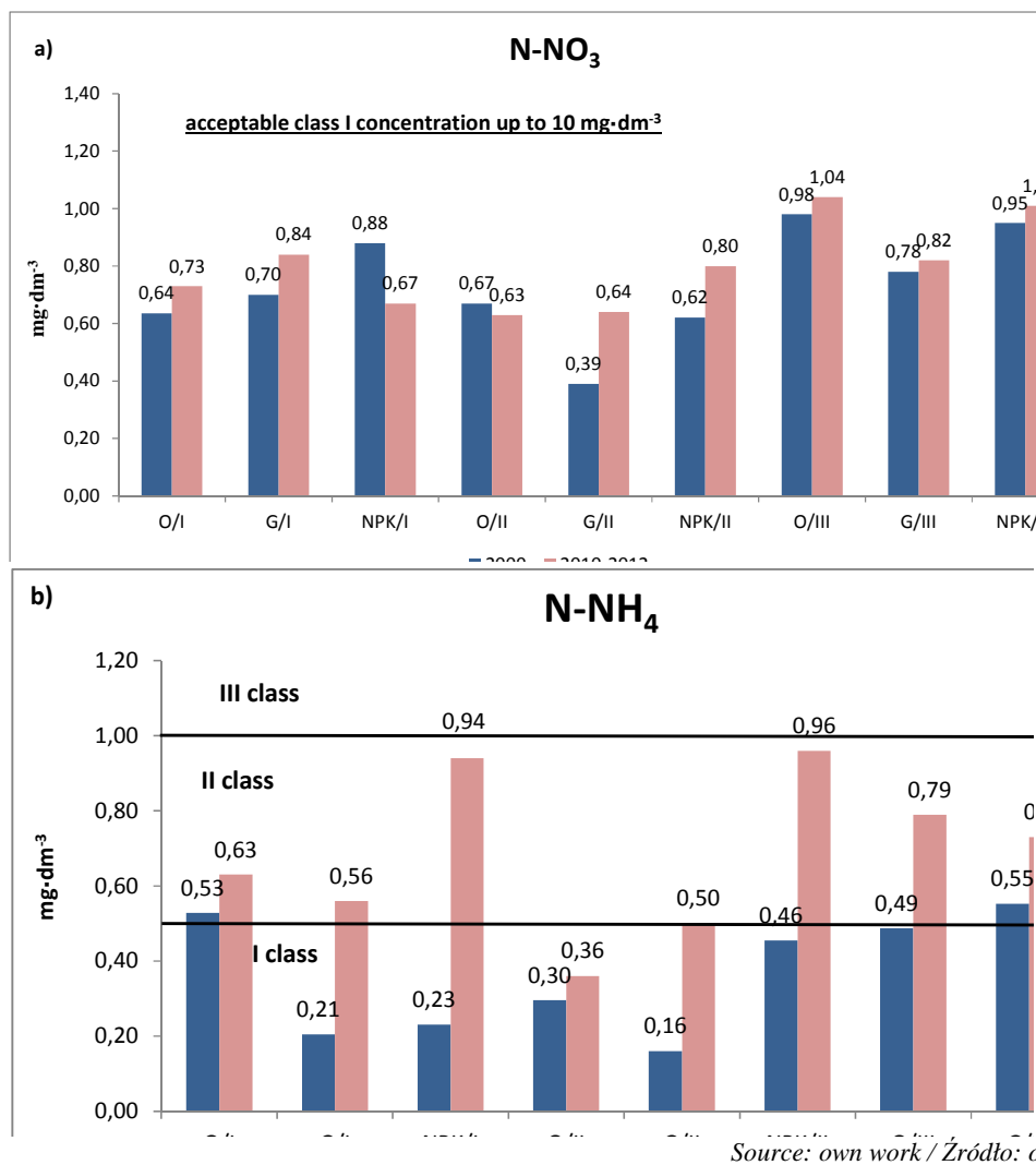
Fig. 2. Mean concentrations of inorganic nitrogen forms during the study period [mg·dm -3 ] Rys. 2. Średnie stężenia mineralnych form azotu za okres badań [mg·dm -3 ]
