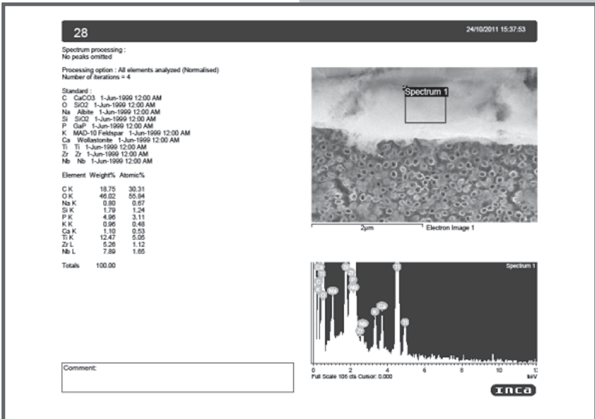
RYS. 2. Analiza EDS dla próbki porowatej Ti13Nb13Zr z naniesioną powłoką HA. FIG. 2. EDS analysis for porous Ti13Nb13Zr with hydroxyapatite layer.
