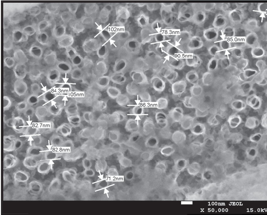
RYS. 1. Powierzchnia stopu Ti13Nb13Zr po utlenianiu i ekspozycji w roztworze Ringera przez okres 28 dni. x50 000. FIG. 1. Porous Ti13Nb13Zr after immersion in Ringer's solution for 28 days, magnification x 50 000.
