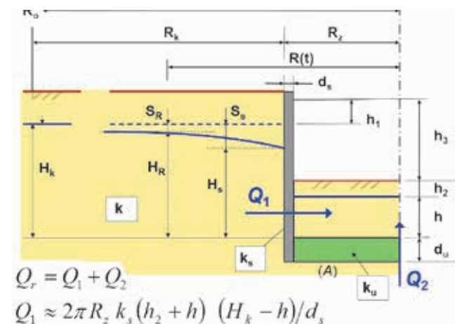
Ryc. 4. Dopływ wody do wykopu
