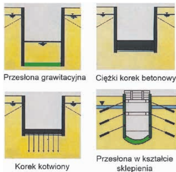
Ryc. 2. Warianty przesłon poziomych
