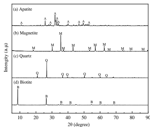
Fig. 1. XRD patterns of (a) apatite, (b) magnetite, (c) quartz, and (d) biotite
