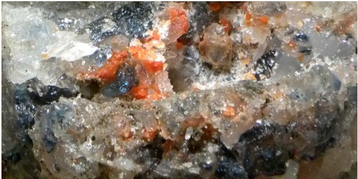
Ryc. 4. Chaotyczna makrotekstura plamistego sylwinitu (rzeczywisty rozmiar w świetle przechodzącym) Fig. 4. Disordely macrotexture of mottled sylvinite (real size in transmitted light)
